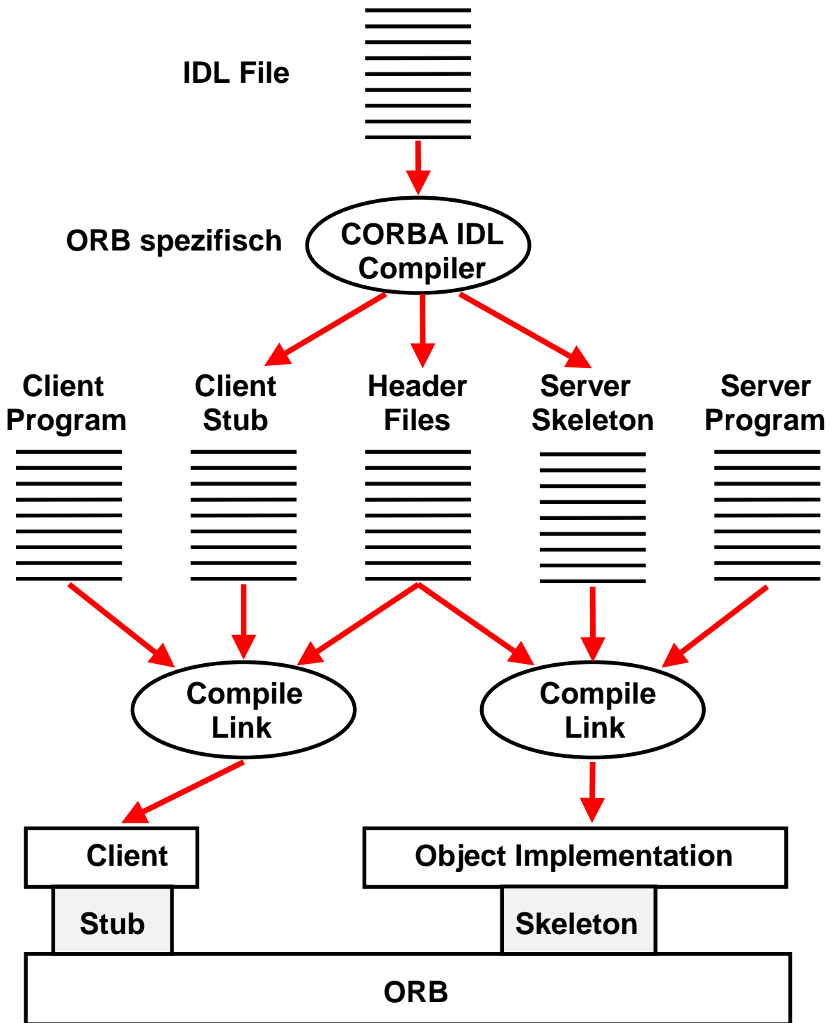
Erstellung von Client und Objekt-Implementation mittels des OMG IDL-Compilers
